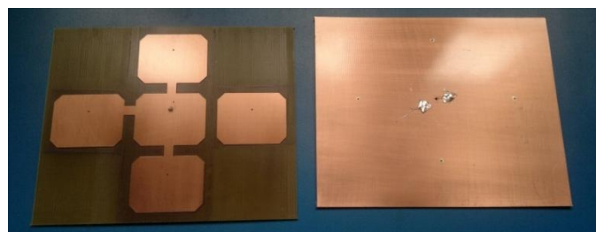
Fig. 10. Prototipo del arreglo de parches rectangulares con cortes y cortos en los parches secundarios.
