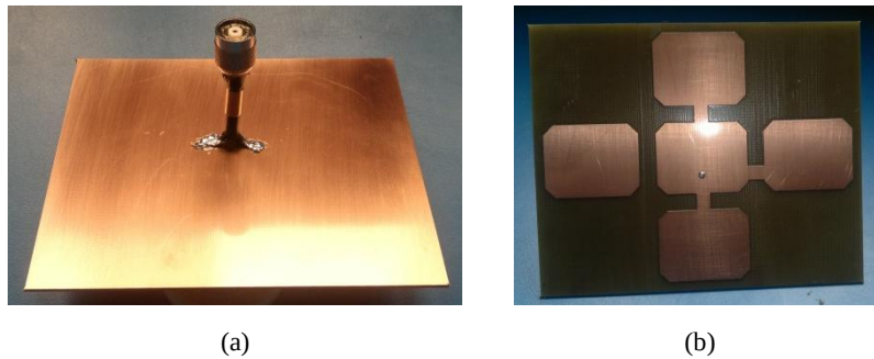
Fig. 11. Prototipo del arreglo de parches rectangulares con cortes, conector de tipo N invertido. Vista: (a) posterior y (b) frontal
