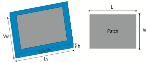
Fig. 2. Dimensiones de una antena de parche rectangular.
