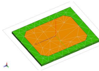
Fig. 4. Antena de parche rectangular con cortes en las esquinas.
