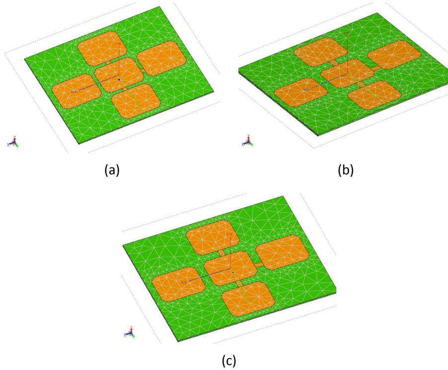
Fig. 5. (a) Arreglo con parches rectangulares con cortes, con una separación de \lambda_g/16 ; (b) arreglo con parches rectangulares con cortes, con una separación de \lambda_g/8 ; (c) arreglo con parches rectangulares con cortes, con una separación de \lambda_g/8 , y cortocircuitos en los parches secundarios.
