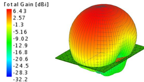
Fig. 6. Patrón de radiación de la ganancia (campo lejano) del Arreglo Rectangular Wi-Fi con cortes_cortos.
