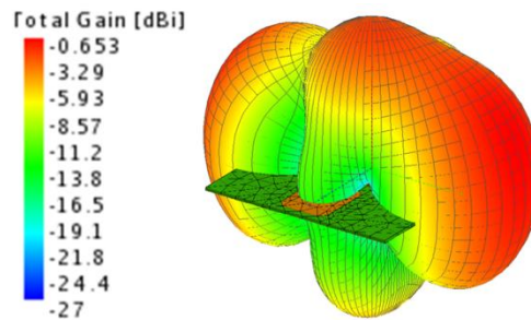
Fig. 7. Patrón de radiación de la ganancia (campo lejano) del Arreglo Rectangular Wi-Fi con cortes.
