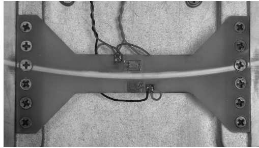
Figura 10. Transductor de fuerza.
