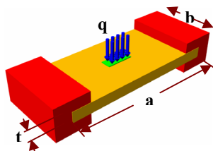
Figura 2. Material, condiciones de carga y empotramientos.
