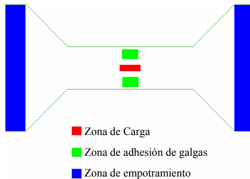
Figura 7. Geometría de la placa en forma de I.
