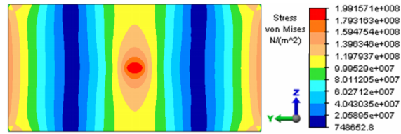
Figura 3. Esfuerzos (Pa) en la placa rectangular de 6 cm de ancho.
