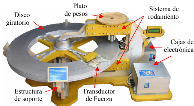
Figura 1. Banco de Pruebas para pesaje dinámico.
