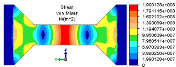
Figura 8. Esfuerzos (Pa) en la placa en forma de I.
