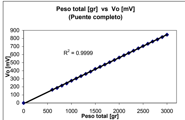
Figura 11. Linealidad del transductor de fuerza. Peso total vs voltaje de salida.
