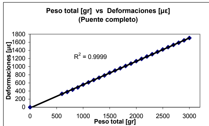
Figura 12. Linealidad del transductor de fuerza. Peso total vs deformaciones unitarias.
