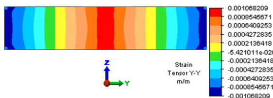
Figura 6. Deformación (m/m) en la placa rectangular de 2.5 cm de ancho.
