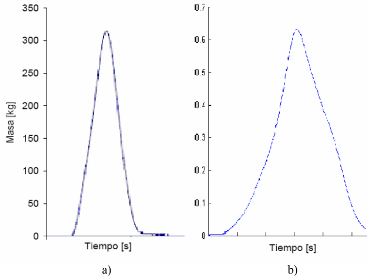
Figura 13. a) Curva dinámica de un prototipo para vehículos ligeros. b) Curva dinámica del banco de pruebas WIM.
