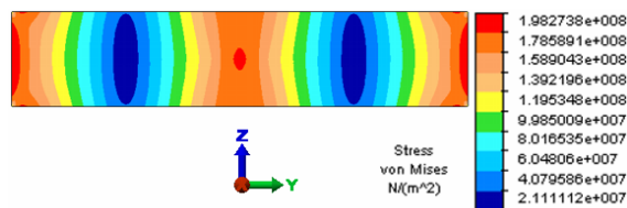
Figura 5. Esfuerzos (Pa) en la placa rectangular de 2.5 cm de ancho.
