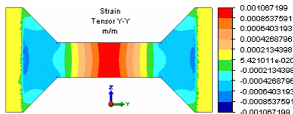
Figura 9. Deformación (m/m) en la placa en forma de I.
