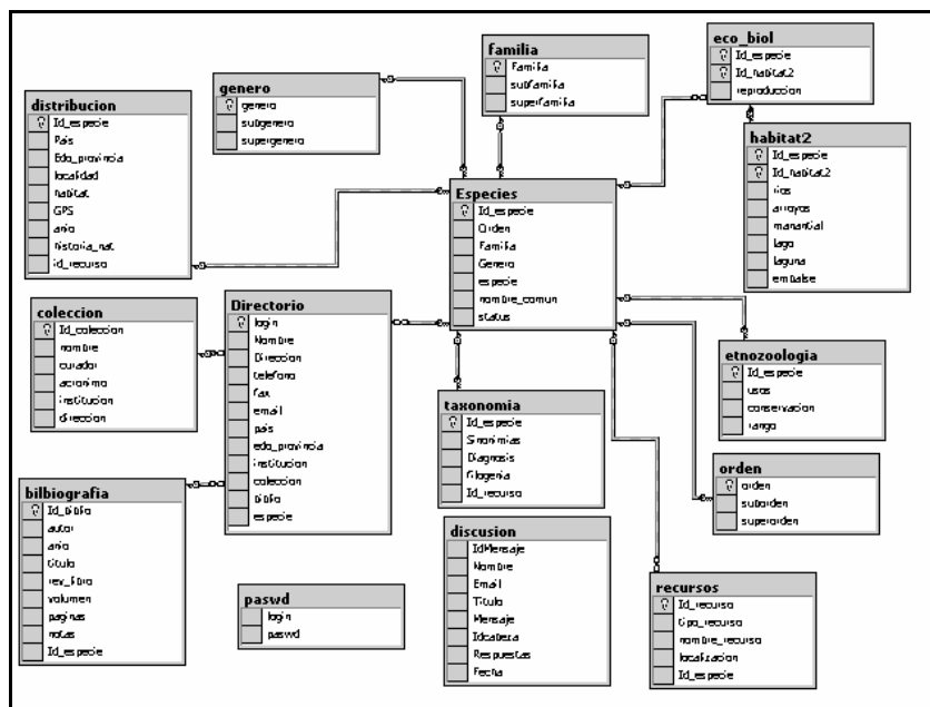
Fig. 2. Diagrama de la base de datos del Sistema Generador de Listados
