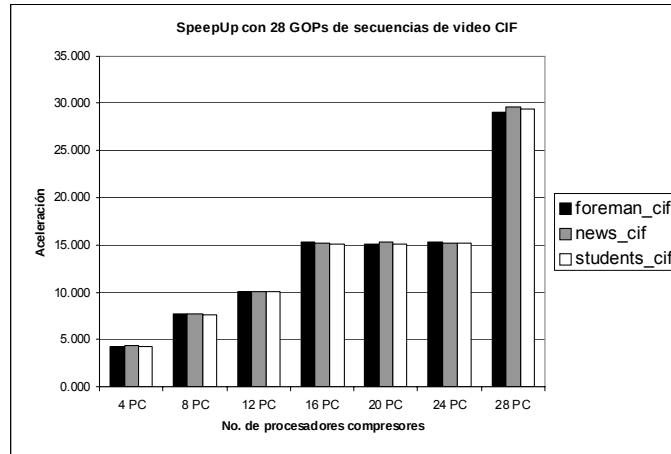
Figura 8 SpeedUp con 28 Gops de secuencias de video CIF
