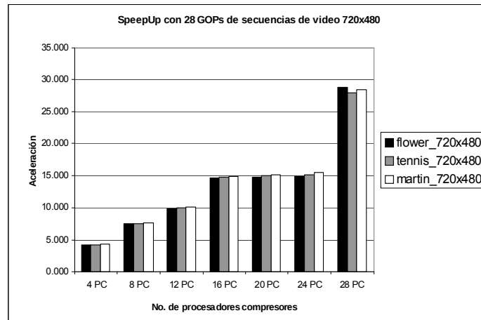
Figura 9 SpeedUp con 28 Gops de secuencias de video 720x480
