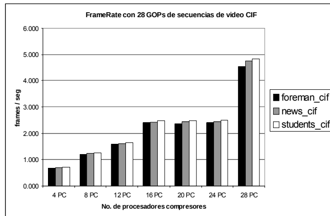
Figura 6 FrameRate con 28 Gops de secuencias de video CIF
